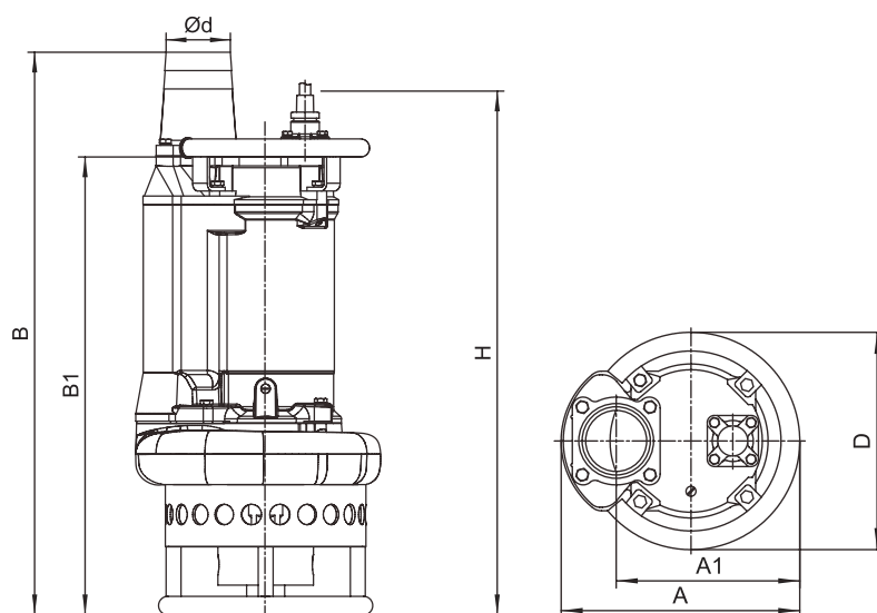
Рисунок 3 – Габаритные и присоединительные размеры насосов серии USP4A
