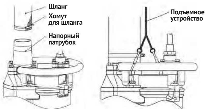
Рисунок 9 – Подключение и перемещение насоса
