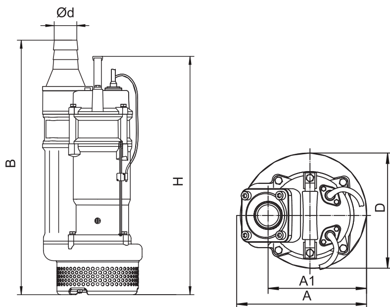
Рисунок 2 – Габаритные и присоединительные размеры насосов серии USPA
